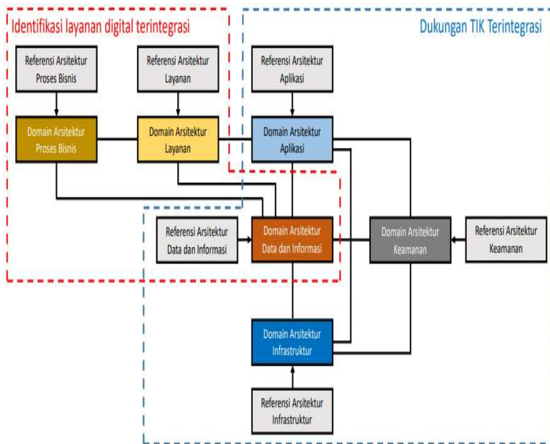
Gambar 6. Keterkaitan Antar Komponen dalam Arsitektur SPBE
